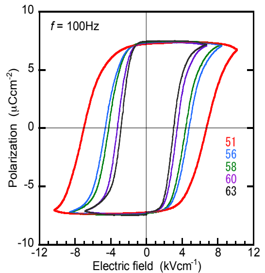
図 1. \text{TTF} \cdot \text{CA} における電場-分極履歴
