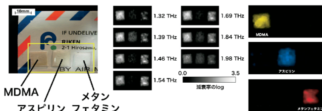
MDMA（麻薬）、アスピリン（頭痛薬）、メタンフェタミン（覚醒剤）を封筒の中に入れたときのテラヘルツ波分光イメージ。指紋スペクトルの違いから封筒内の試薬の空間分布が得られる 1) 。
